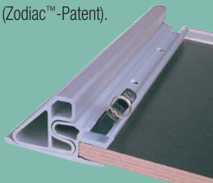
Marinesperrholzboden mit Aluminiumrahmen und integrierten Profilschienen.
